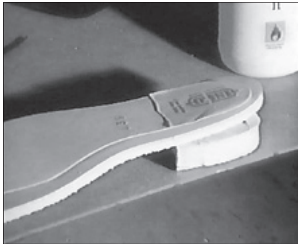
Irralliset sisäpohja ja ulkopohja, joiden väliin päällisnahen reunat tulevat, sekä kengän kanta.
